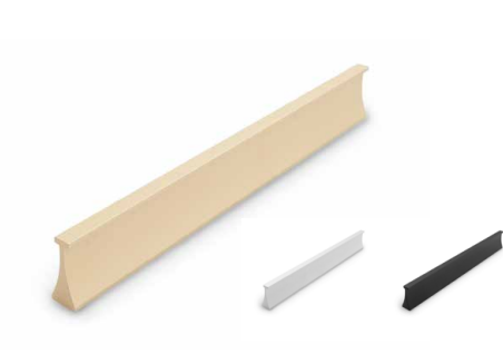
Профиль-ручка 180 мм Материал: алюминий Размеры: 180x23x10 мм
