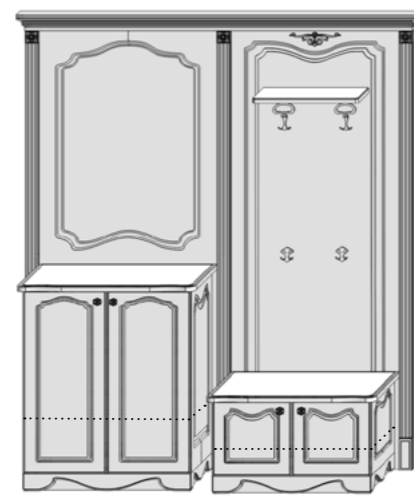
Vers.kit.hall-2 □ 1882 □ 2156 □ 496
