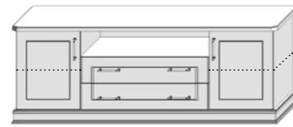
Yv.TTV-1 □ 1562 □ 575 □ 490
