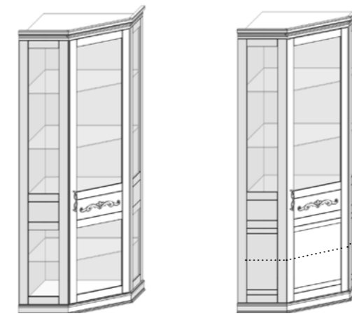
Avi.PU-1 751 2156 751 Avi.PU-2 751 2156 751
