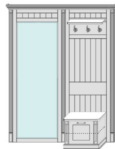
Yv.kit.hall-3 □ 1362 □ 2156 □ 496
