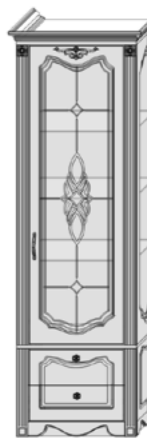
Vers.PV.1S.O-5 □ 698 □ 2156 □ 504
