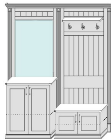
Yv.kit.hall-2 □ 1882 □ 2156 □ 496
