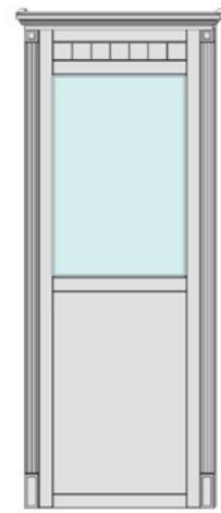
Yv.2.SPO.(z).SRED □ 744 □ 2156 □ 64 □ 874 □ 2156 □ 64 □ 1004 □ 2156 □ 64 □ 1134 □ 2156 □ 64
