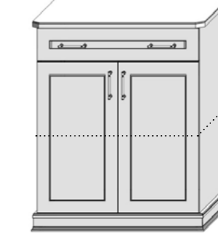
Yv.TPR-V4 □ 806 □ 971 □ 430
